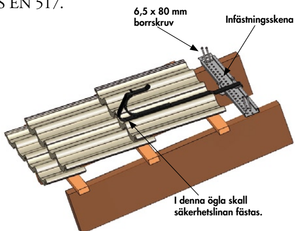
Bild 2. Montering av infästningsskena.
