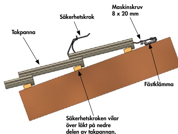
Bild 3. Montering av säkerhetskrok i infästningsskena.
