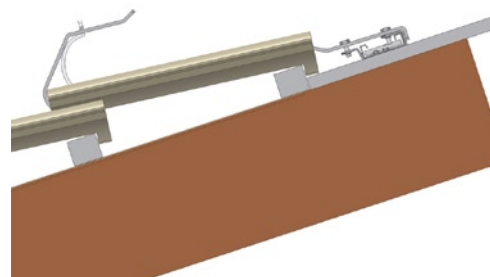
Bild 4. Vid 45 mm läkt skall en 22 mm läkt läggas under skenan på takstolen där skenan fästes.
